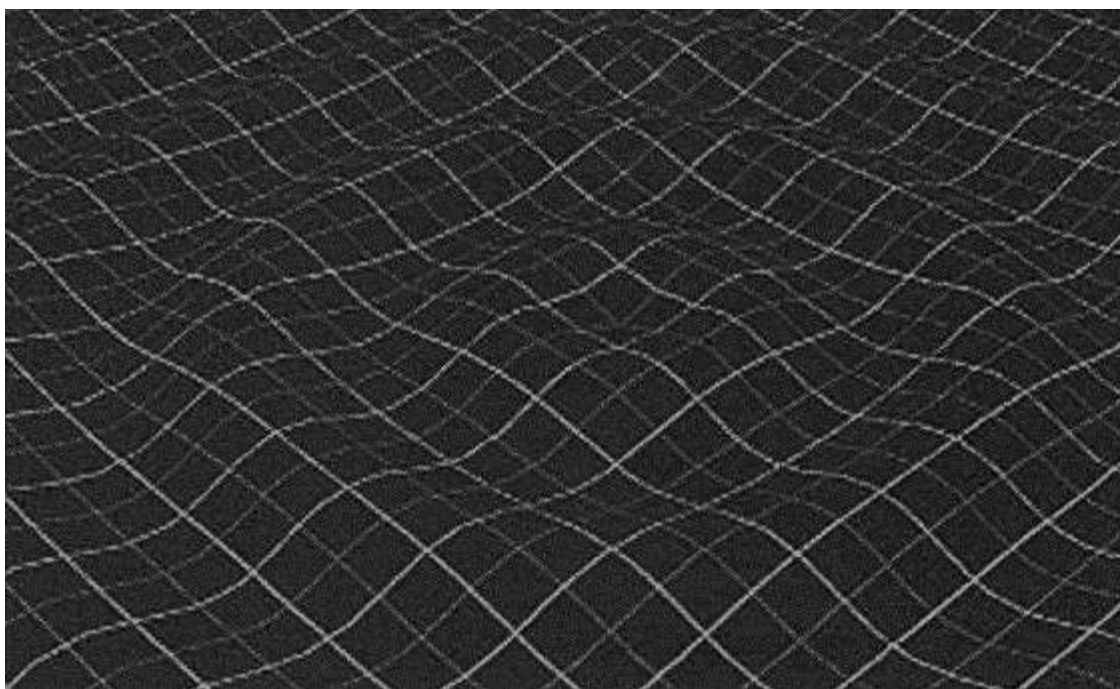
Thí dụ sóng hấp dẫn như sóng gợn trong tấm vải không-thời-gian (Courtesy of Brian Greene)
