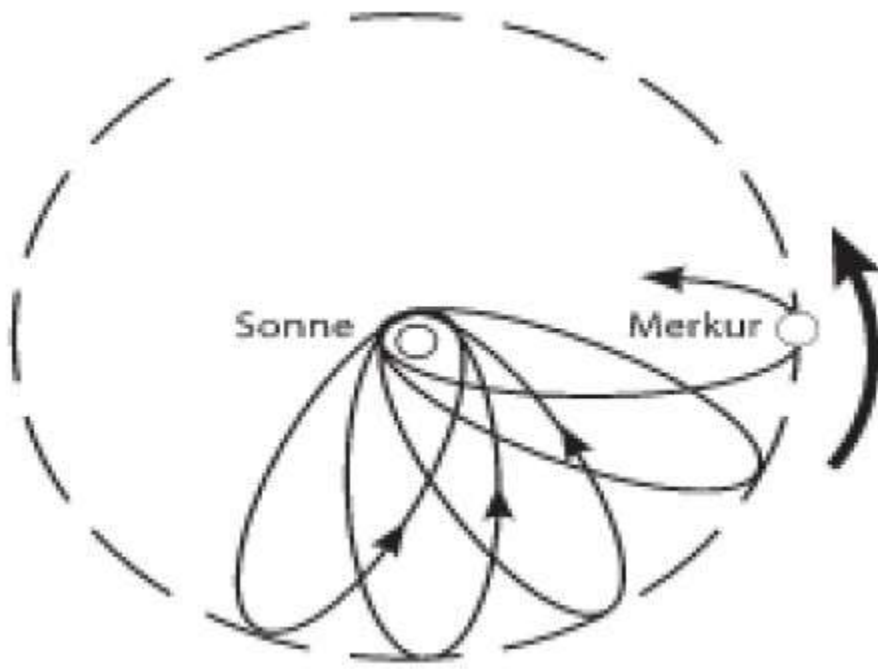
Quỹ đạo của sao Mercury (sao Thủy)
