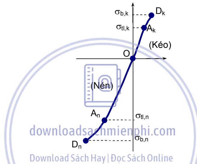
Hình 3.5. Quan hệ ứng suất – biến dạng trong thí nghiệm kéo và nén vật liệu dẻo
