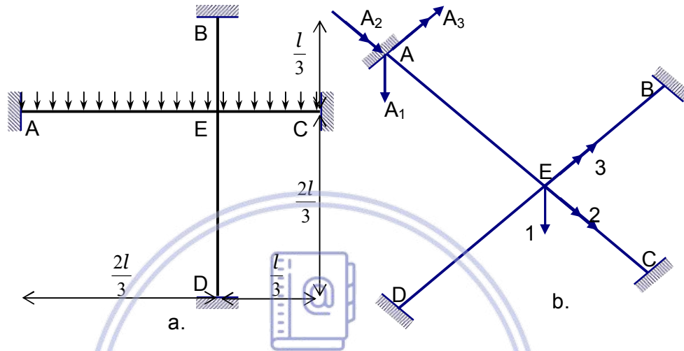
Hình 12.7. Khung ngang
