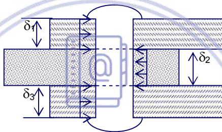
Hình 6.10. Kiểm tra ứng suất ép tại các mặt tiếp xúc
