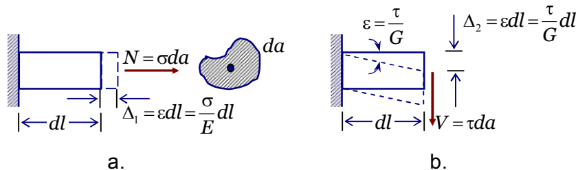
Hình 3.1. Phần tử thanh
