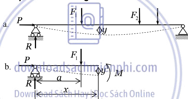
Hình 9.4. Thanh chịu uốn ngang và uốn dọc đồng thời
