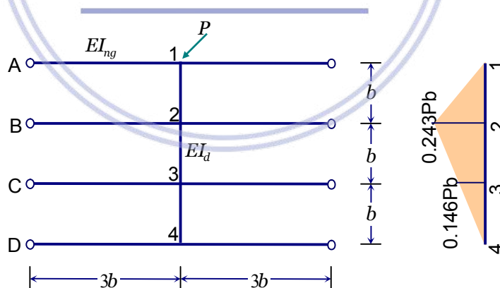
Hình 12.11. Hệ khung ngang và biểu đồ nội lực
