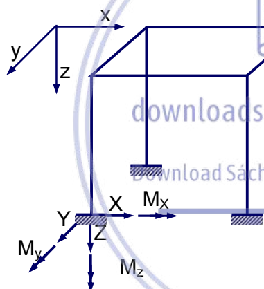
Hình 10.4. Hệ khung không gian
