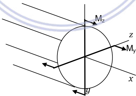
Hình 8.4. Thanh chịu uốn xiên
