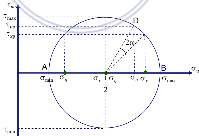
Hình 2.7. Đường tròn Mohr của trạng thái ứng suất phẳng
