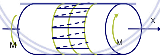
Hình 6.3. Giả thiết về biến dạng khi thanh chịu xoắn
